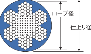
断面図(ビニコート6×19)
