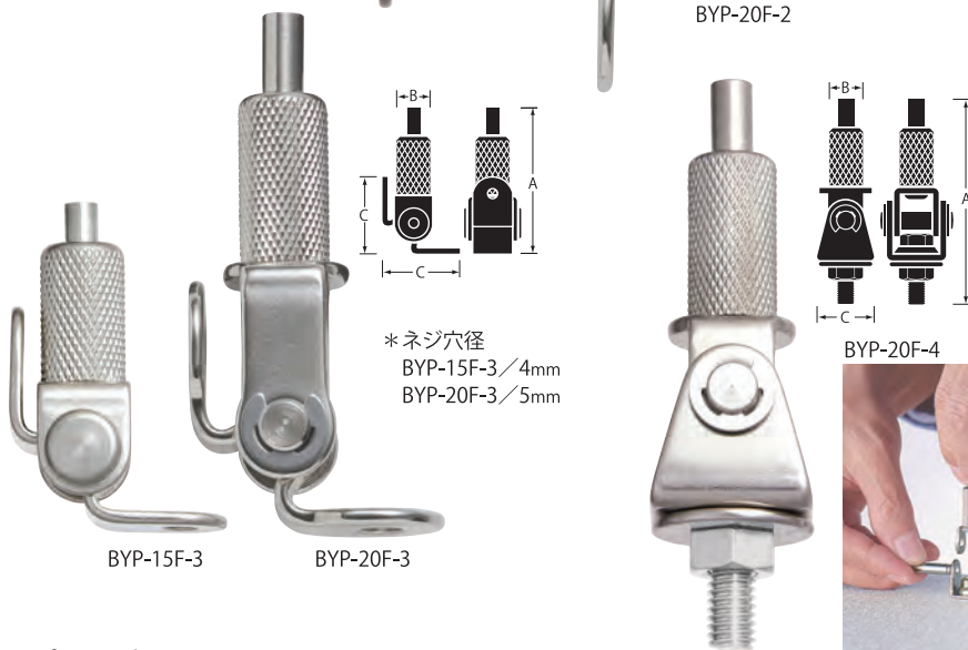
◆角度可動式 可動式の本体部の角度は自由に変えられます。
