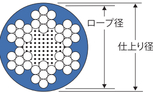
断面図(ビニコート6×7)
