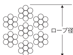
断面図(7×7)
