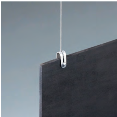
M4ボルト付、適合板厚8mm以下。 穴位置(センター) はプレートの端から13mm 以内です。
