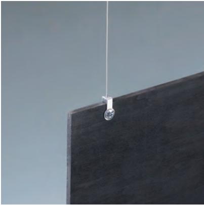
M4ボルト付、適合板厚6mm以下。 穴位置(センター) はプレートの端から10mm 以内です。
