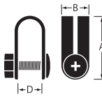
M4ボルト付、適合板厚8mm以下。 穴位置(センター) はプレートの端から13mm 以内です。
