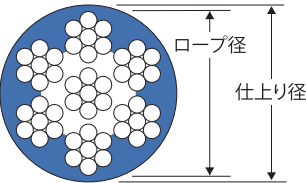
断面図(ビニコート7×7)
