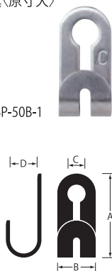
製品写真〈原寸大〉
